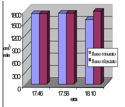
Fig. 2 – Confronto tra i flussi rilasciati e i flussi misurati nel corso di uno dei test del sistema
