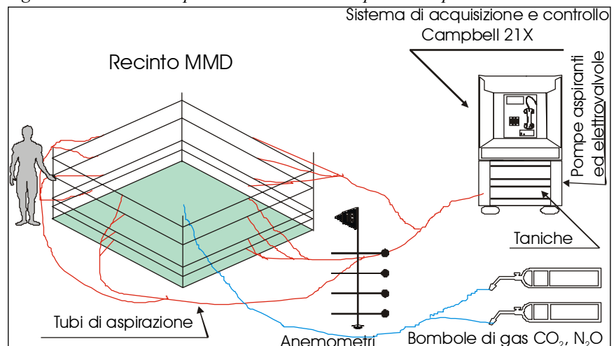
Fig. 1 - Schema dell'impianto MMD realizzato presso l'Ispaim CNR
